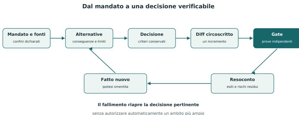
Figura 6.1 — Il prompt avvia un ciclo di comprensione, scelta, modifica e verifica; un fallimento riapre la decisione senza allargare automaticamente l’ambito.
