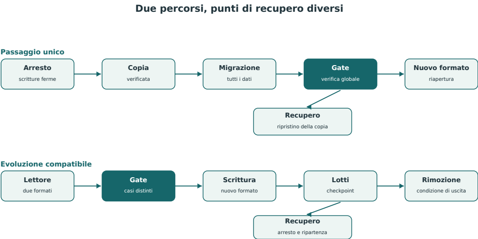
Figura 7.1 — La migrazione immediata concentra trasformazione e recupero; l’evoluzione compatibile introduce gate e checkpoint lungo il percorso.
