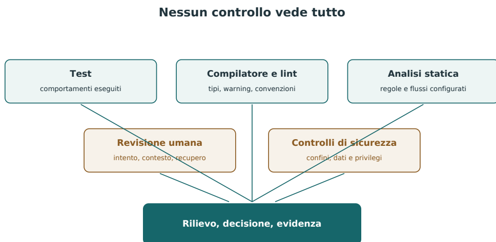
Figura 14.1 — Test, compilatore, analisi, revisione umana e controlli di sicurezza osservano parti diverse. Il risultato utile è un rilievo collegato a decisione ed evidenza.
