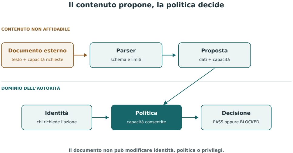
Figura 17.1 — Il contenuto attraversa un parser con schema dichiarato e può soltanto proporre dati e capacità. La politica, l'identità e il contesto operativo restano fuori dal contenuto; soltanto il valutatore produce la decisione.
