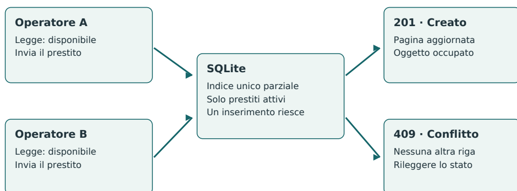
Figura T.2 — Due letture possono indicare disponibile. Soltanto una scrittura ottiene il prestito: il database impedisce la seconda riga attiva, mentre la pagina spiega il conflitto.
