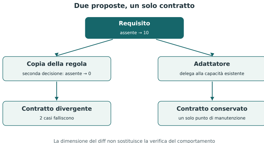
Figura 8.2 — Il confronto riguarda il contratto: la copia introduce una seconda decisione sul valore mancante, il riuso mantiene la regola condivisa e lascia locale soltanto l'adattamento.
