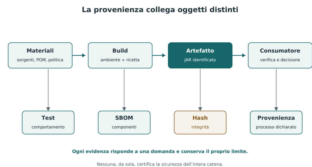
Figura 17.2 — La provenienza collega materiali, ricetta, ambiente e artefatto. Le evidenze restano distinte: una SBOM descrive componenti, un test osserva comportamento e un hash rileva differenze.
