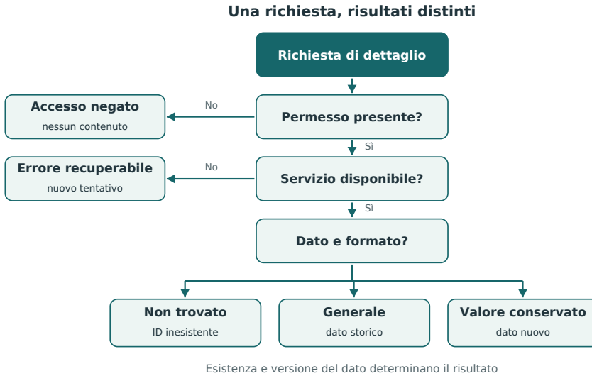
Figura 4.2 — Permesso, disponibilità, esistenza e versione del dato conducono a risultati distinti; un unico valore di ripiego cancellerebbe informazioni necessarie.
