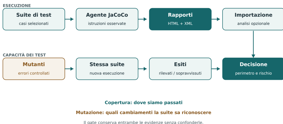
Figura 15.1 — La copertura registra le parti attraversate; il mutation testing verifica se la suite distingue alcune modifiche del comportamento. I due risultati rispondono a domande diverse e confluiscono nella stessa decisione tracciata.
