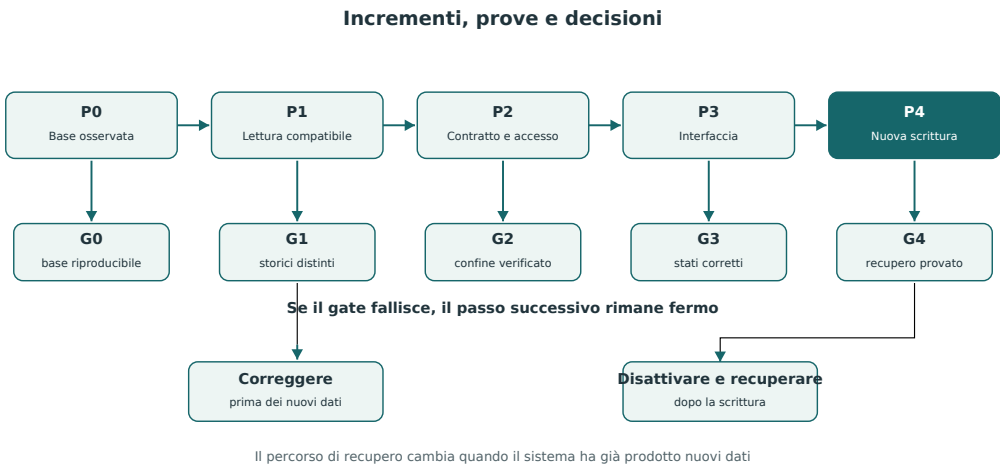
Figura 5.1 — Ogni incremento produce un comportamento osservabile e incontra un punto di decisione; il recupero cambia quando la modifica ha già prodotto nuovi dati.
