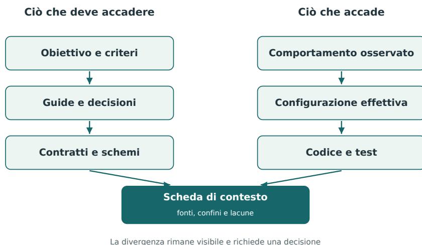
Figura 3.1 — La scheda di contesto confronta fonti normative e descrittive; una divergenza diventa una lacuna da risolvere, non un dettaglio da nascondere.
