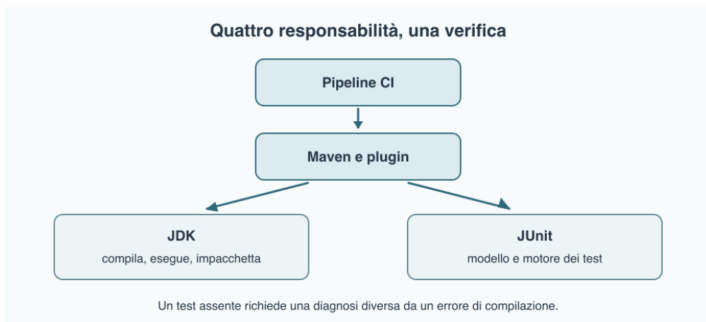
Figura 29.2 – La pipeline avvia la build; Maven orchestra plugin e dipendenze; il JDK compila ed esegue; JUnit definisce e lancia i test attraverso la piattaforma.
