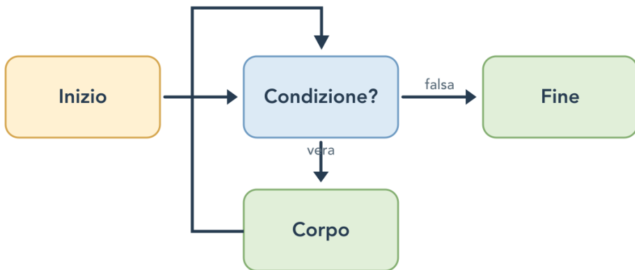
Figura 5.1 – Il corpo viene ripetuto finché la condizione è vera. La freccia di ritorno porta alla verifica, non direttamente al corpo.
