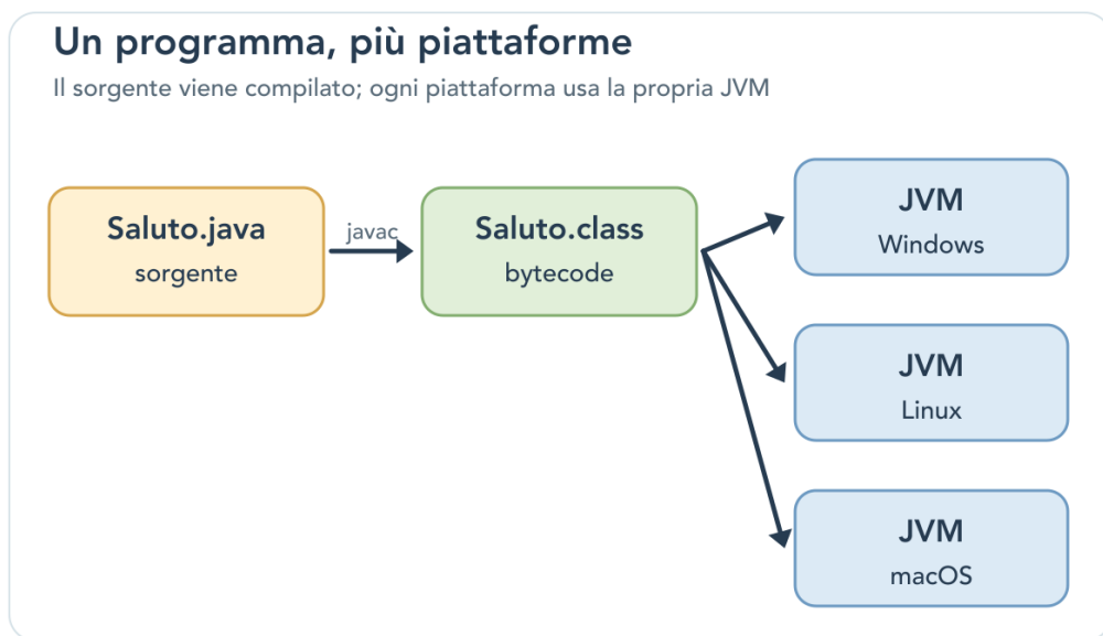
Figura 3.2 – Il bytecode consente a JVM per piattaforme diverse di eseguire il programma. Il file sorgente viene compilato una volta nell'esempio; ciascuna piattaforma dispone del proprio ambiente di esecuzione.
