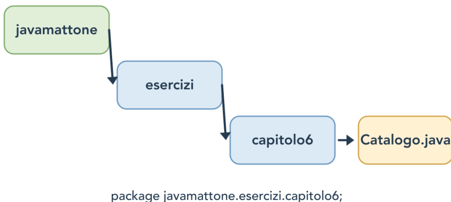
Figura 6.1 – Il nome del package e la gerarchia dei sorgenti si corrispondono nel nostro progetto. La classe Catalogo è collocata nella cartella finale.
