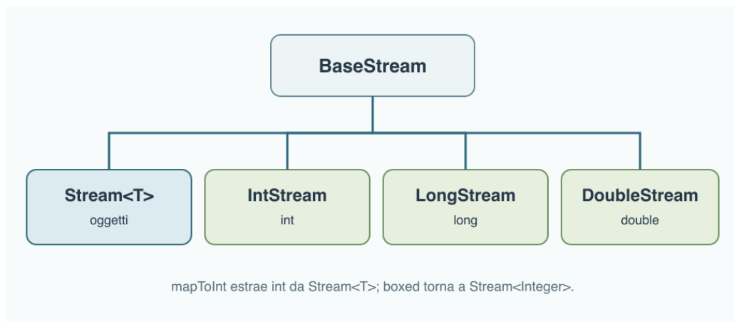
Figura 18.3 - Stream<T> elabora oggetti; IntStream, LongStream e DoubleStream elaborano i tre primitivi supportati dalle API specializzate.
