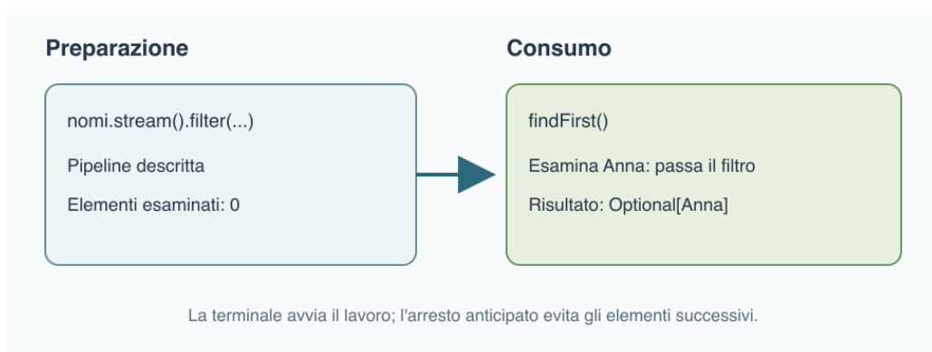
Figura 18.2 – Costruire filter non visita i nomi; findFirst avvia la ricerca e può fermarla sul primo risultato.
