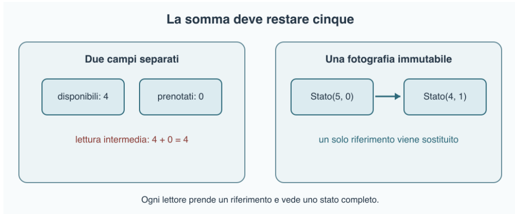
Figura 20A.3 – Un riferimento atomico a uno stato immutabile pubblica insieme i valori collegati, a condizione che tutti i lettori usino la stessa fotografia.
