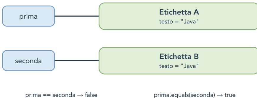
Figura 10.1 - Due etichette diverse possono avere lo stesso valore. Un codice hash uguale è richiesto per oggetti uguali; da solo non prova che gli oggetti siano uguali.
