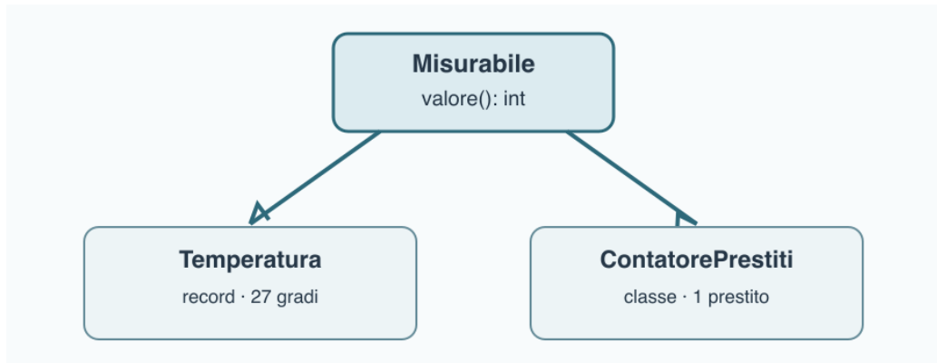
Figura 13.1 – Un'interfaccia permette di chiedere valore() a oggetti non imparentati per classe. Temperatura e ContatorePrestiti possono anche implementare Descrivibile senza rinunciare alla loro diversa struttura interna.
