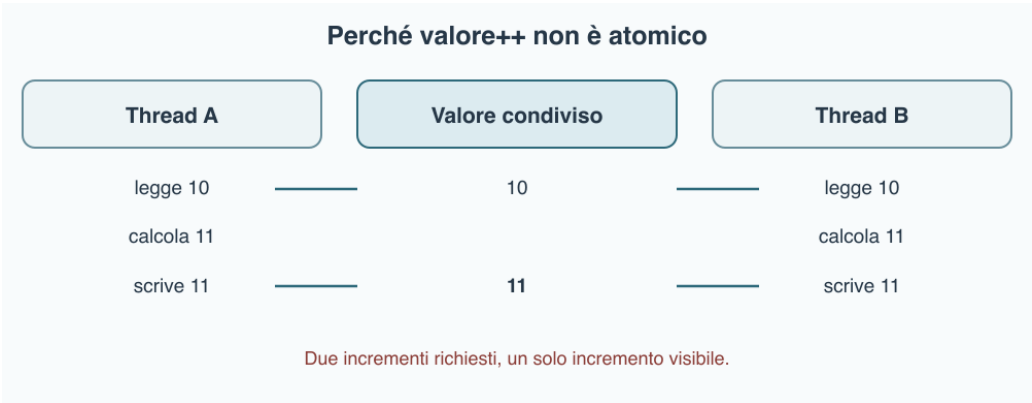
Figura 20.5 - Due letture dello stesso valore prima delle scritture producono un incremento perso.
