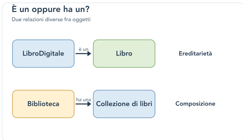
Figura 2.5 – «È un» e «ha una» portano a scelte diverse. LibroDigitale può essere un tipo di Libro ; una Biblioteca ha una collezione di libri, ma non è una collezione di libri.
