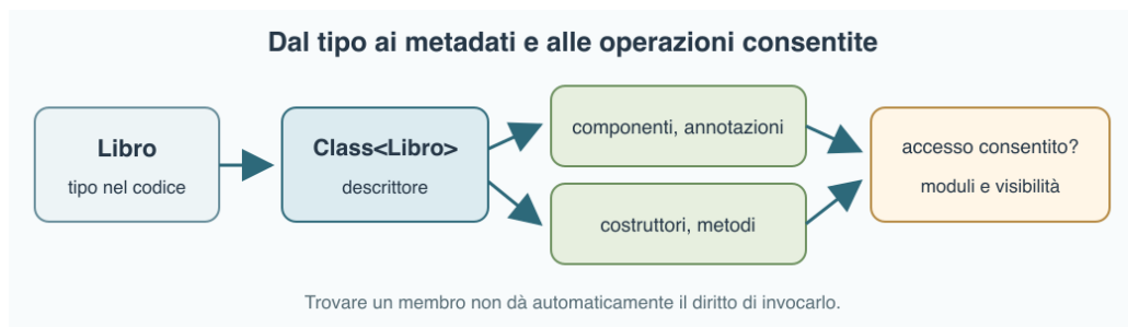
Figura 24.1 – Ispezione e invocazione sono passi distinti; l'accesso segue le regole del linguaggio e dei moduli.
