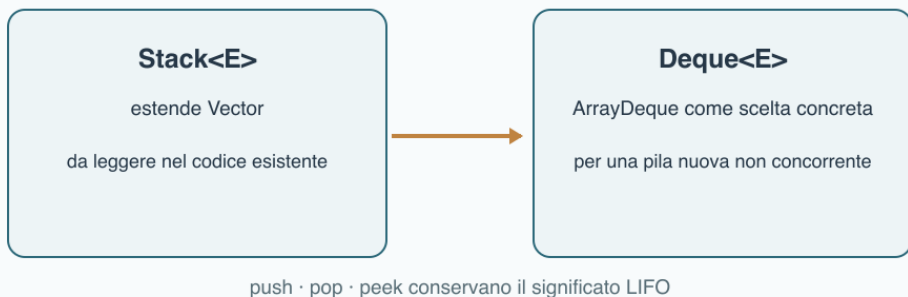
Figura 17.5 – Il comportamento LIFO resta lo stesso; nel codice nuovo Deque esprime meglio la scelta della struttura. ArrayDeque è una possibile implementazione non concorrente.
