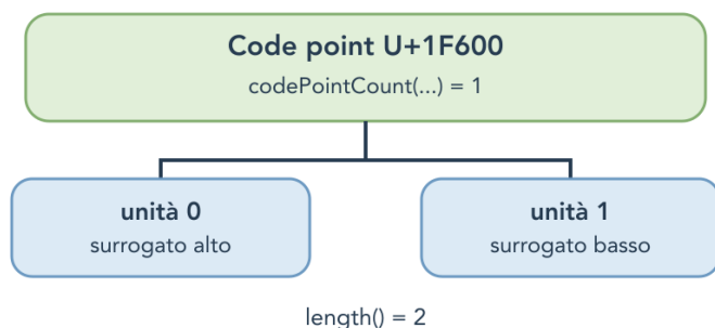
Figura 11.2 – Il simbolo dell'esempio occupa due posizioni UTF-16. length() restituisce 2; codePointCount(0, length()) restituisce 1.
