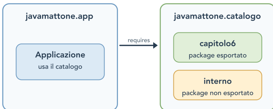
Figura 6.3 – javamattone.app legge javamattone.catalogo , che esporta il package del capitolo 6. Il nome capitolo6 nella figura abbrevia javamattone.esercizi.capitolo6 ; il package interno rappresenta un'eventuale parte non esportata. Un semplice import non renderebbe accessibile quella parte dall'applicazione esterna.
