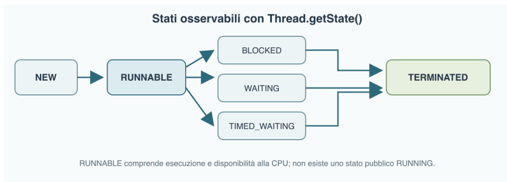
Figura 20.4 – Stati e transizioni principali di Thread.
