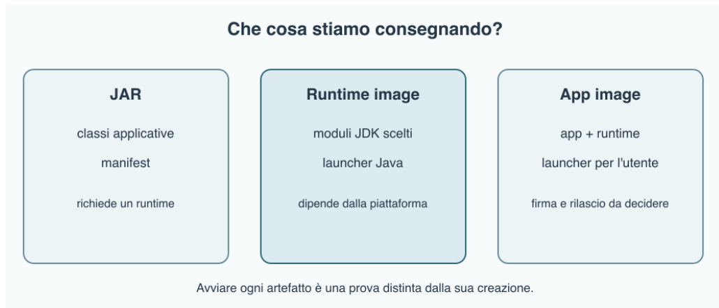
Figura 29.3 – Il JAR porta l'applicazione, il runtime image porta i moduli JDK scelti, il pacchetto riunisce ciò che serve all'utente della piattaforma di destinazione.
