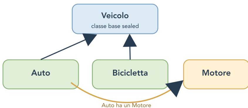
Figura 9.1 – Auto e Bicicletta sono specializzazioni di Veicolo ; Auto contiene un Motore . Le frecce delle sottoclassi puntano alla classe base. Il collegamento con il motore indica una parte, non un altro tipo di veicolo.
