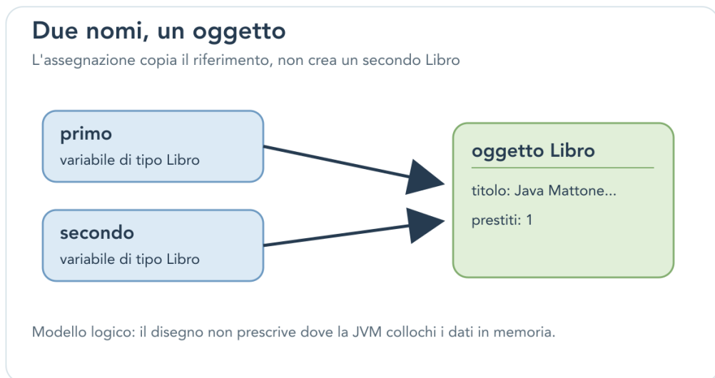
Figura 7.1 – primo e secondo indicano la stessa istanza di Libro . La figura è un modello logico dei riferimenti: non prescrive in quale area fisica della memoria la JVM debba collocare i dati.
