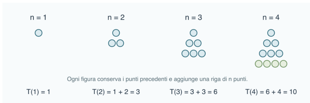
Figura 16.2 – Per ottenere T(n) si conservano i punti di T(n - 1) e si aggiunge una riga di n punti. Il colore diverso dell'ultima riga del quarto disegno mostra il passo ricorsivo.
