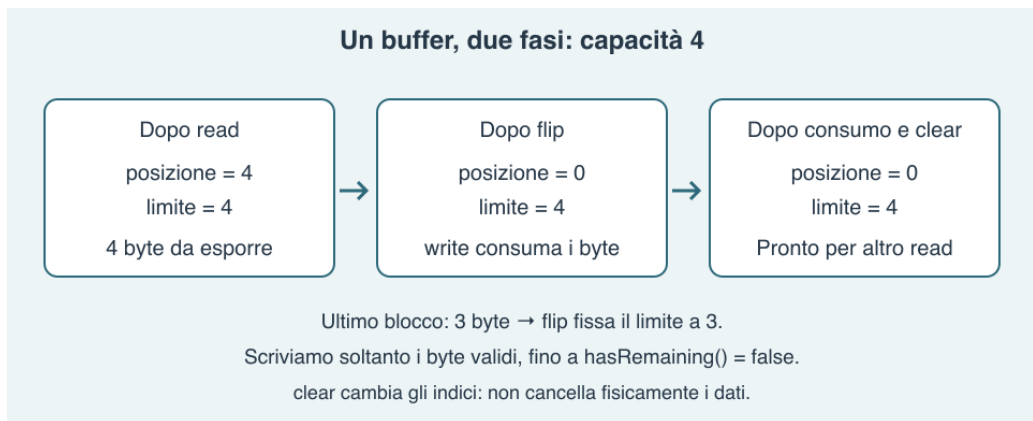
Figura 25.3 – Posizione e limite delimitano i byte validi durante la copia.
