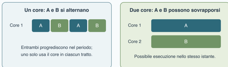
Figura 20.2 - Due possibili esecuzioni: i riquadri non promettono turni fissi. La priorità non determina l'ordine del programma.
