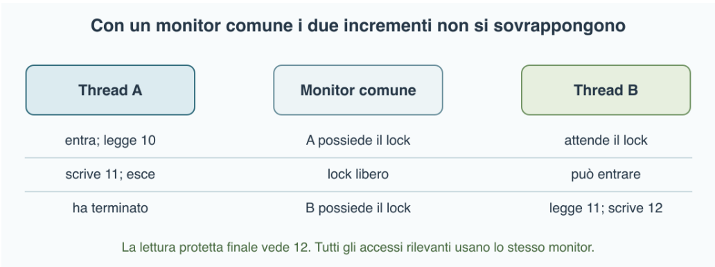
Figura 20.6 - La vista accoppiata alla figura precedente: con lo stesso monitor la seconda lettura avviene dopo la prima scrittura.
