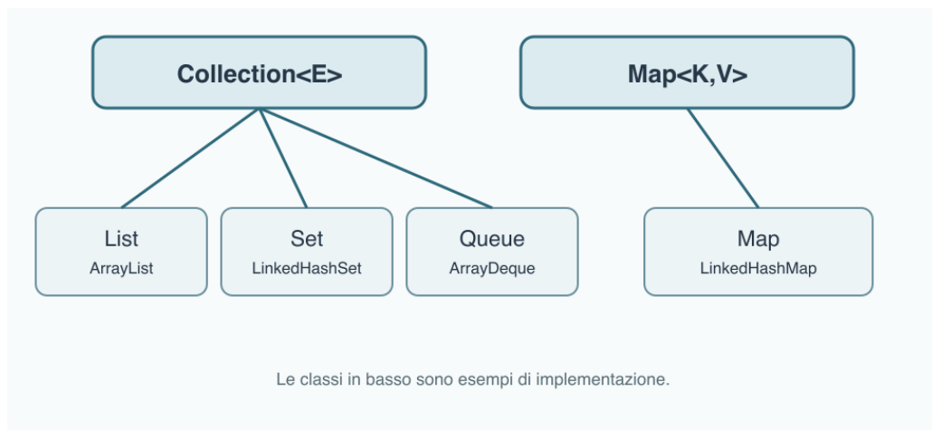
Figura 17.1 – Collection e Map rispondono a esigenze diverse. Le interfacce dichiarano il contratto; classi come ArrayList , LinkedHashSet e LinkedHashMap sono scelte concrete con proprietà proprie.
