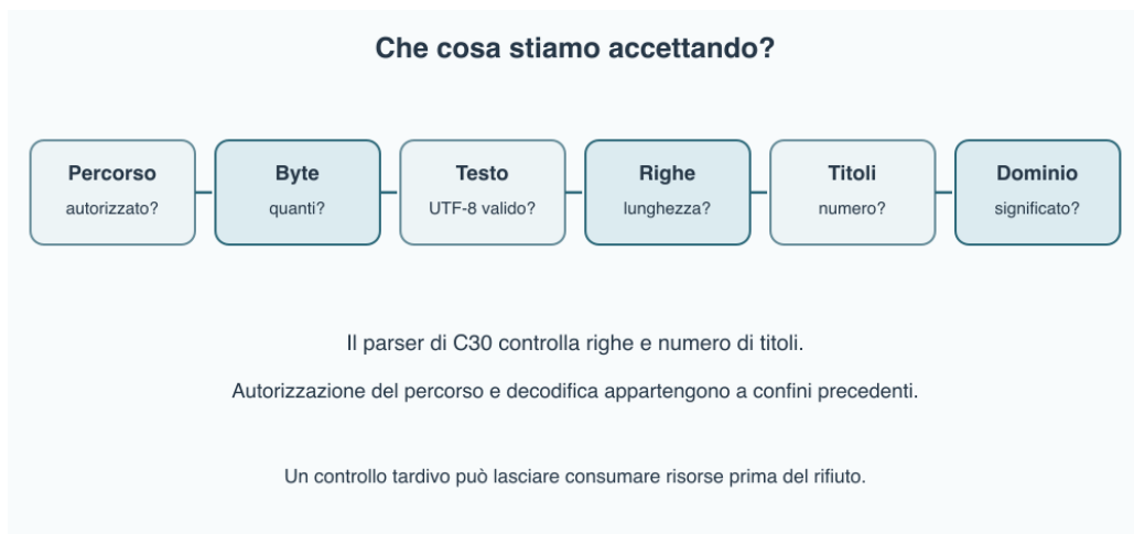
Figura 30.2 – La validazione segue l'ingresso dal nome del file fino alla regola di dominio; ciascun passaggio ha rischi e limiti propri.
