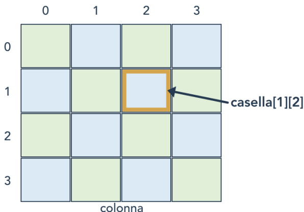
Figura 4.2 – La casella caselle[1][2] è nella seconda riga e nella terza colonna. La figura mostra una griglia regolare; Java permette anche righe di lunghezze diverse.
