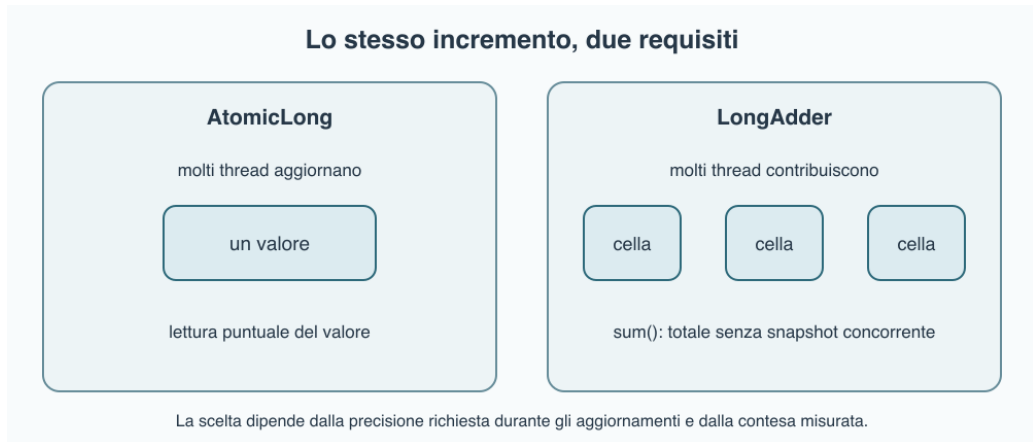
Figura 20A.2 – Un adder raccoglie contributi distribuiti: sum() durante gli aggiornamenti non è una fotografia atomica del totale.
