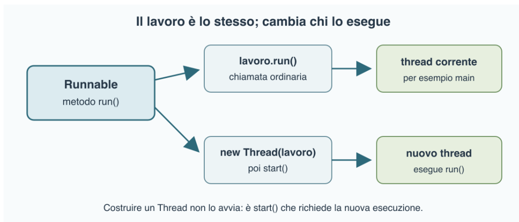
Figura 20.3 – run() chiamato direttamente resta nel chiamante; start() richiede un nuovo thread che eseguirà lo stesso lavoro.
