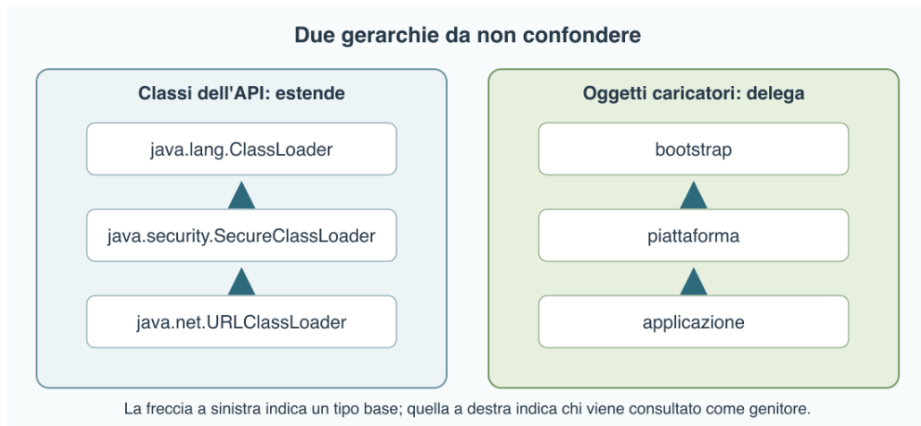
Figura 21.3 – A sinistra un esempio di ereditarietà pubblica verificabile nell'API; a destra la relazione di delega tipica dei caricatori integrati.
