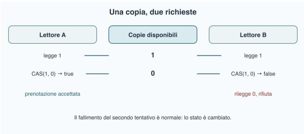
Figura 20A.1 – Due lettori possono osservare «1», ma uno solo può sostituirlo con «0» quando il confronto e la sostituzione costituiscono un'unica operazione.
