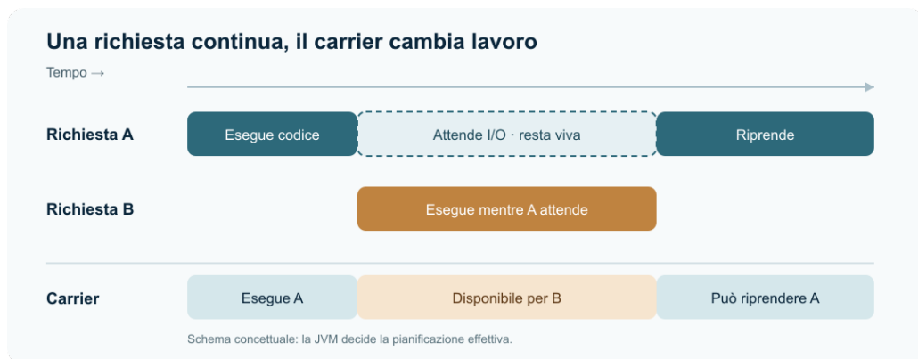
Figura 20.10 – Un thread virtuale rappresenta la richiesta per tutta la sua durata; il carrier è occupato soltanto mentre ne esegue il codice. Quando la richiesta A attende l'I/O, la JVM può usare lo stesso carrier per la richiesta B. La figura rappresenta il meccanismo, non una sequenza temporale garantita dal programma.
