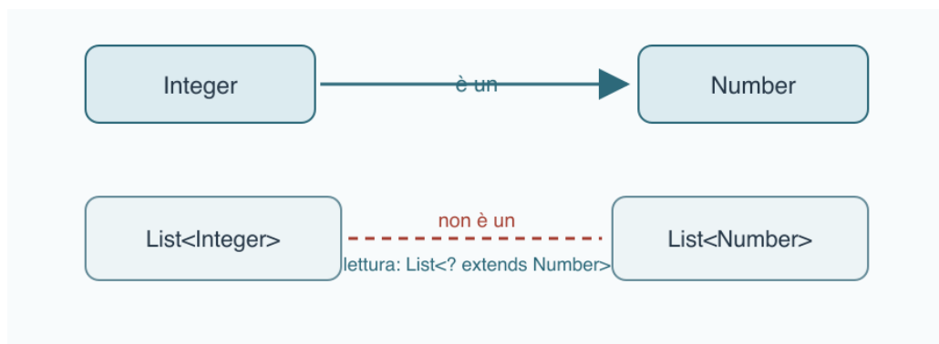
Figura 15.1 - Integer è un sottotipo di Number , ma List<Integer> non è un sottotipo di List<Number> . La wildcard descrive la variazione ammessa dal singolo metodo.
