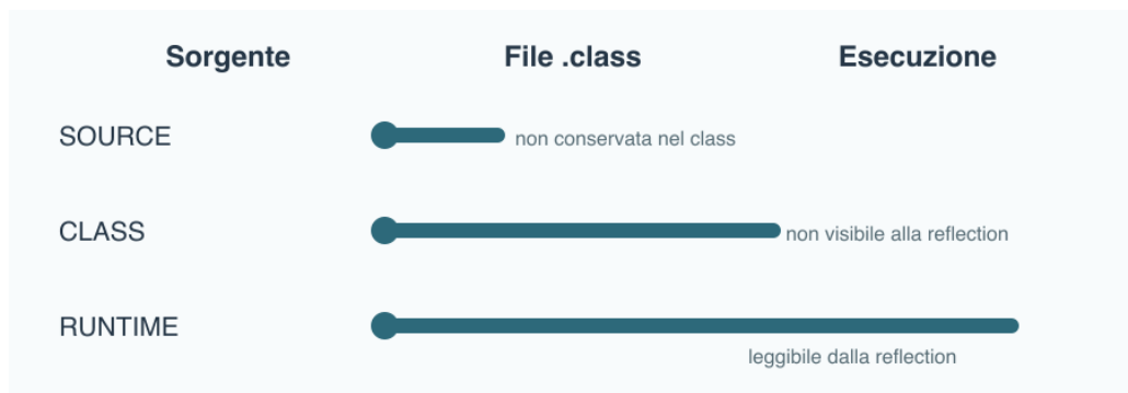
Figura 14.1 – SOURCE, CLASS e RUNTIME indicano fino a quale fase arriva un'annotazione. La politica non decide da sola quale lavoro verrà compiuto su quei metadati.
