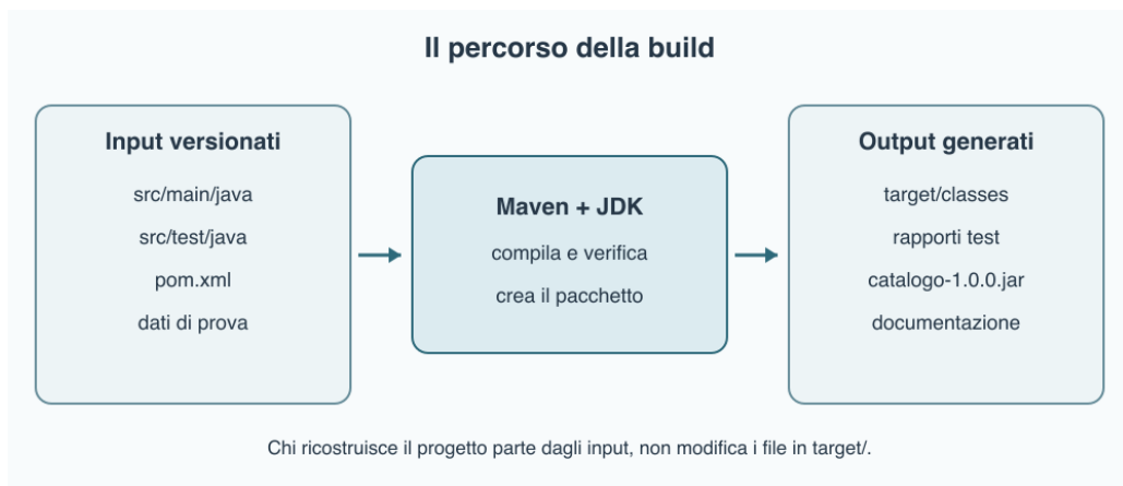
Figura 29.1 – Sorgenti, test e configurazione sono input versionati; classi, rapporti e JAR sono output della build.
