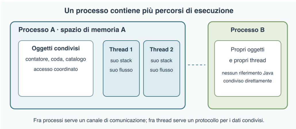
Figura 20.1 – I thread condividono gli oggetti del loro processo, ma mantengono percorsi di esecuzione distinti. I processi hanno spazi separati.
