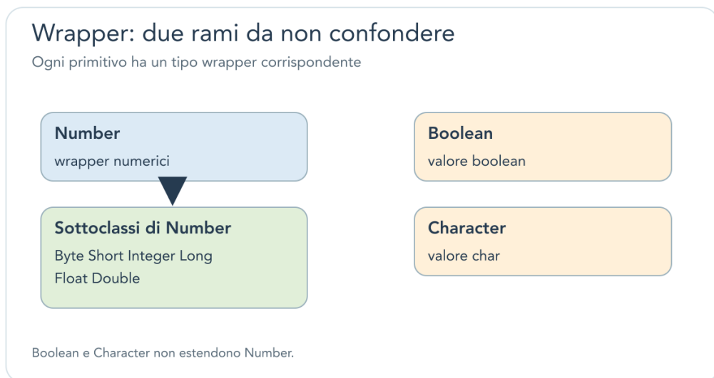
Figura 10.2 – Boolean e Character non sono sottoclassi di Number . Ogni primitivo ha un wrapper, ma la gerarchia delle classi non coincide con una graduatoria di conversioni numeriche.
