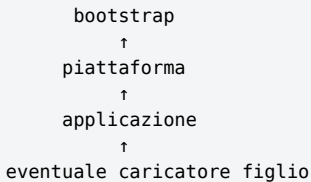
Figura 21.1 – Relazione di delega tipica. La freccia punta verso il genitore consultato prima dal figlio. Non rappresenta ereditarietà fra le classi caricate. Un caricatore personalizzato può scegliere comportamenti speciali; la figura descrive il modello predefinito che studiamo qui.
