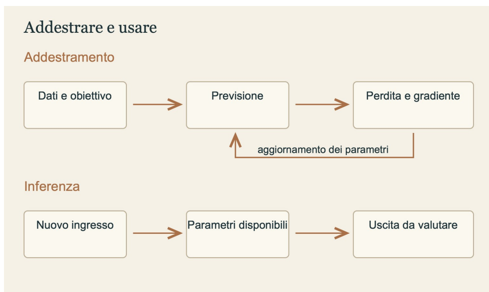
Figura 2 · Addestrare e usare una rete sono processi distinti
