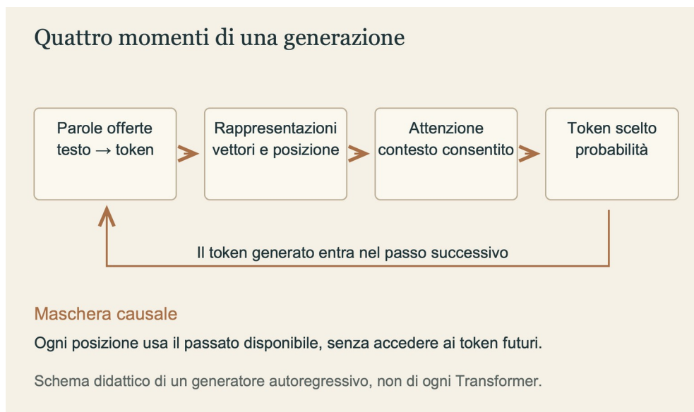
Figura 3 · Quattro momenti di una generazione
